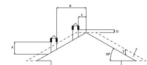
TETTO A 30°
